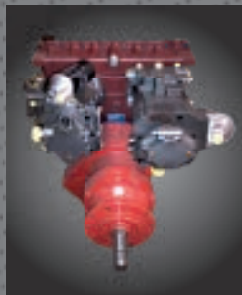
Trasmissione standard sulle coclee per la gamma RE.
