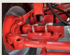
Biasse a bilanciere con assale posteriore sterzante
