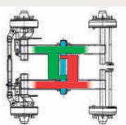
Biasse a bilanciere con assale posteriore sterzante
