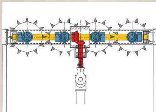
Spanditore con riduttore incorporato versione monotrave di serie su tutta la gamma.
